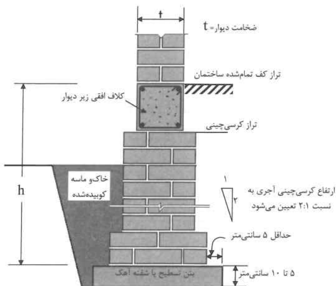
شکل ۶-۷ شالوده متشکل از مجموع کلاف افقی زیر دیوار و کرسه چینی آجر چینی
